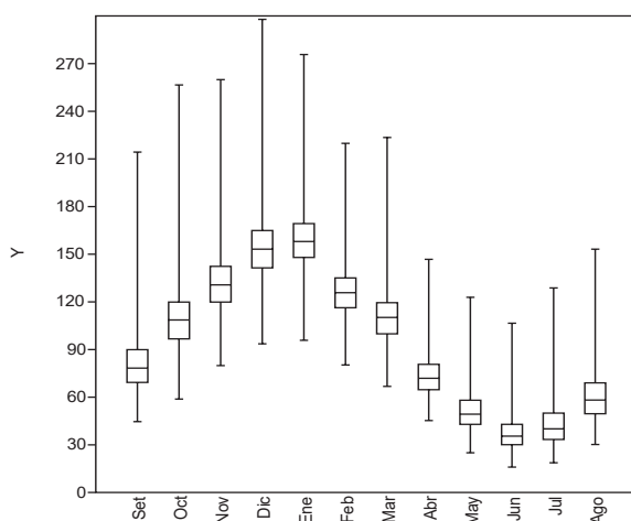
Fig. 10. ETP mensual. Período 1970-2010.
