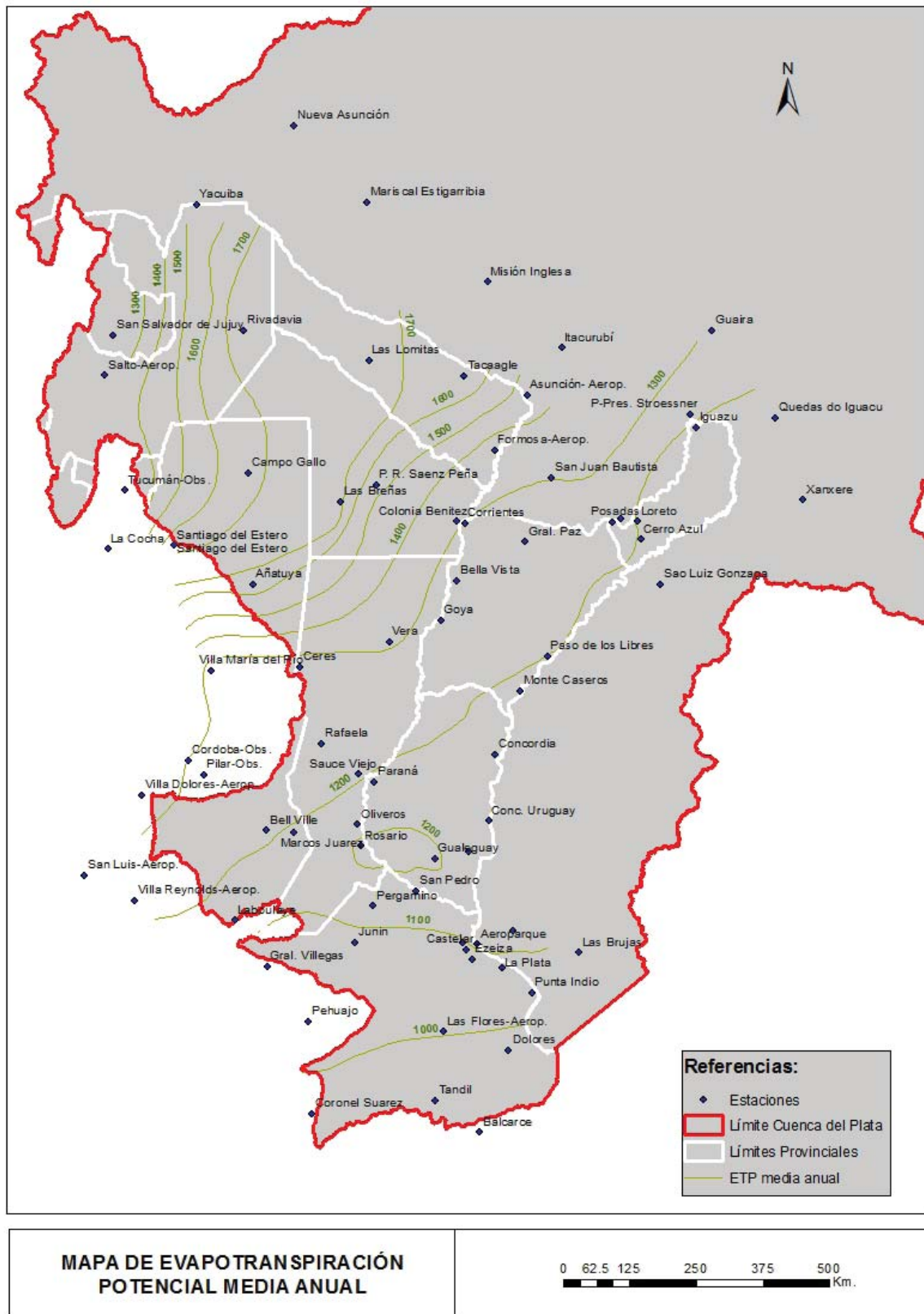
Fig. 9. Isolíneas de ETP medias anuales zona de estudio. Período 1970-2010
